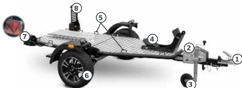
1 - Kupplungskugel, 2 - Mechanismus zum Absenken / Anheben des Anhängers, 3 - Stützrad, 4 - Vorderradbefestigungsrinne, 5 - Befestigungshaken, 6 - Rad (Alufelge als Option), 7 - LED-Heckleuchten, 8 - Kennzeichenhalter
